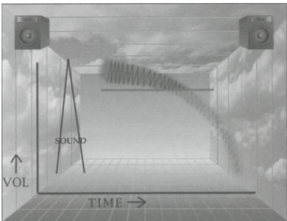
Рис. 106. Огибающая загейтованного реверба.
