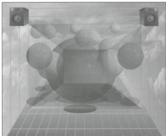
Рис. 219. Удаленный микс.
