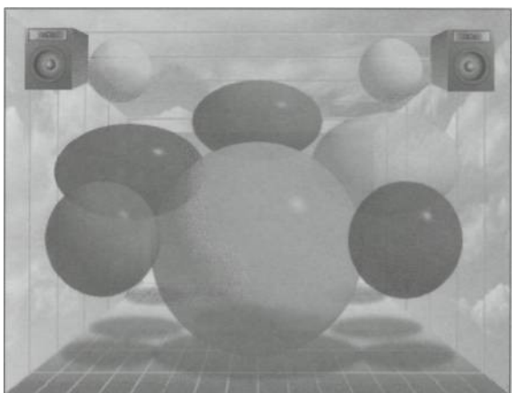
Рис. 194. Сбалансированный микс.
