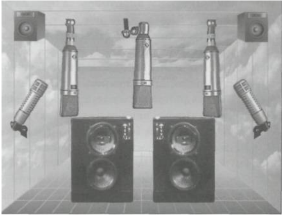
Рис. 54. Преобразователи звука.
