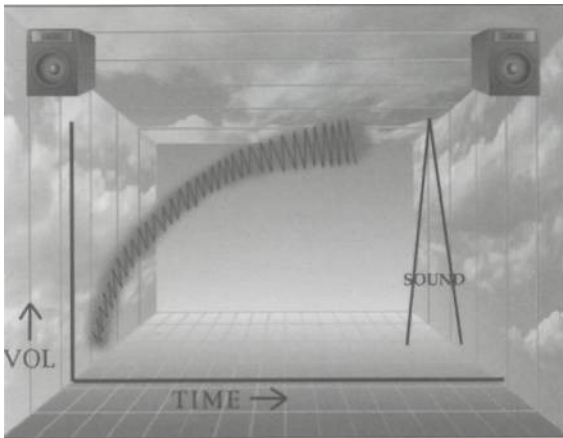
Рис. 108. Преверб.
