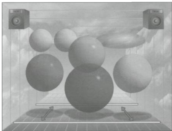
Рис. 42. Ровная громкость
