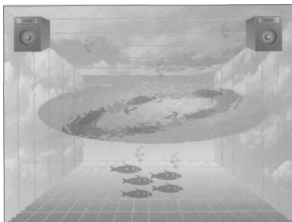
Рис. 209. «Подводный» флейнджер.
