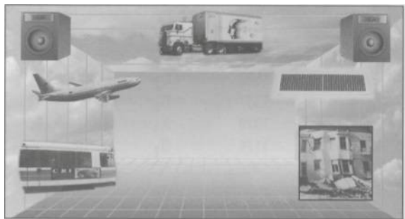
Рис. 73. Источники шума.
