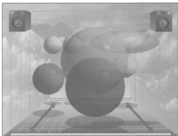
Рис. 43. Неровная громкость.
