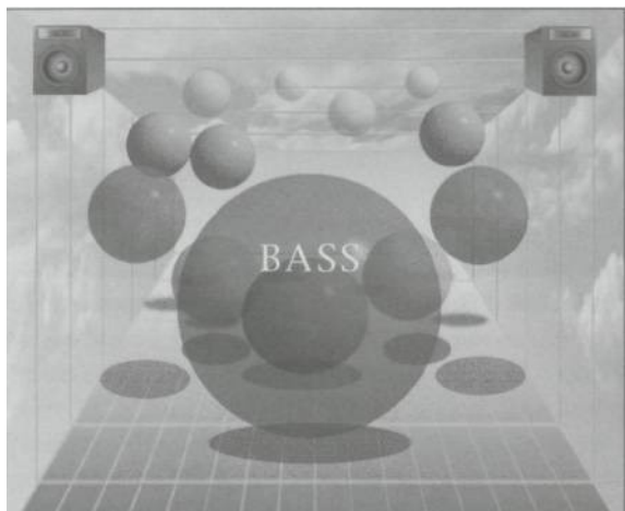
Рис. 184. Панорамирование басгитары.
