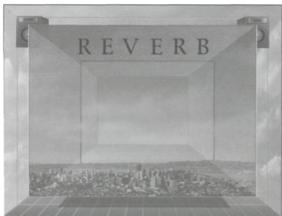
Рис. 207. Пространственный реверб.
