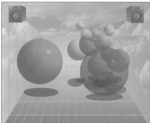
Рис. 195. Смещенный микс.
