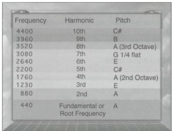
Рис. 76. Гармоническая структура ноты «А» акустической гитары.
