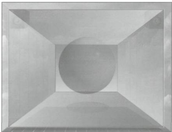
Рис. 39. Громкий реверб.
