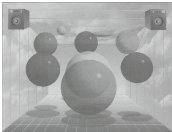
Рис. 48. Разреженный микс.
