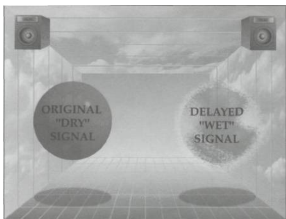
Рис. 208. «Мечтательная» задержка
