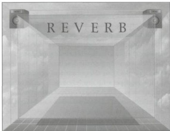
Рис. 213. реверб.
